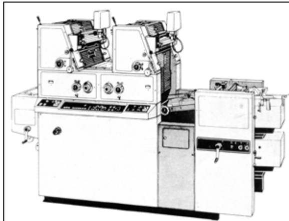
So ungefähr könnte unsere neue Druckmaschine aussehen, für die unsere treuen Leser und Sponsoren seit einem ¼ Jahr gespendet haben.
